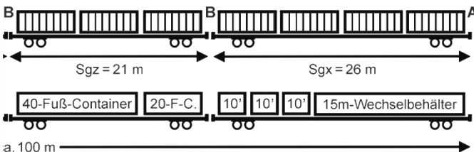
Abb.32: Beispiel für die Zusammenstellung der Güterwagen in einer „CEC-Standardgruppe“. (Zeichenerklärung siehe Tabelle 9)
