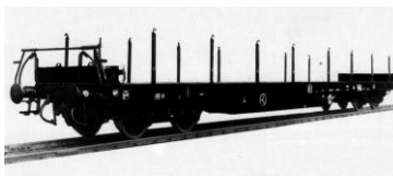
Abb.3: Flachwagen der Baureihe R. Speziell für den Containertransport gebaute Wagen haben zur Gewichtsersparnis auch keine Rungen mehr.
